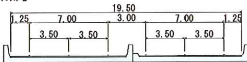
▲標準横断面 (単位：m)
